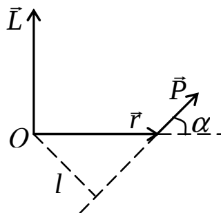
Рисунок 4.1 – Момент импульса
